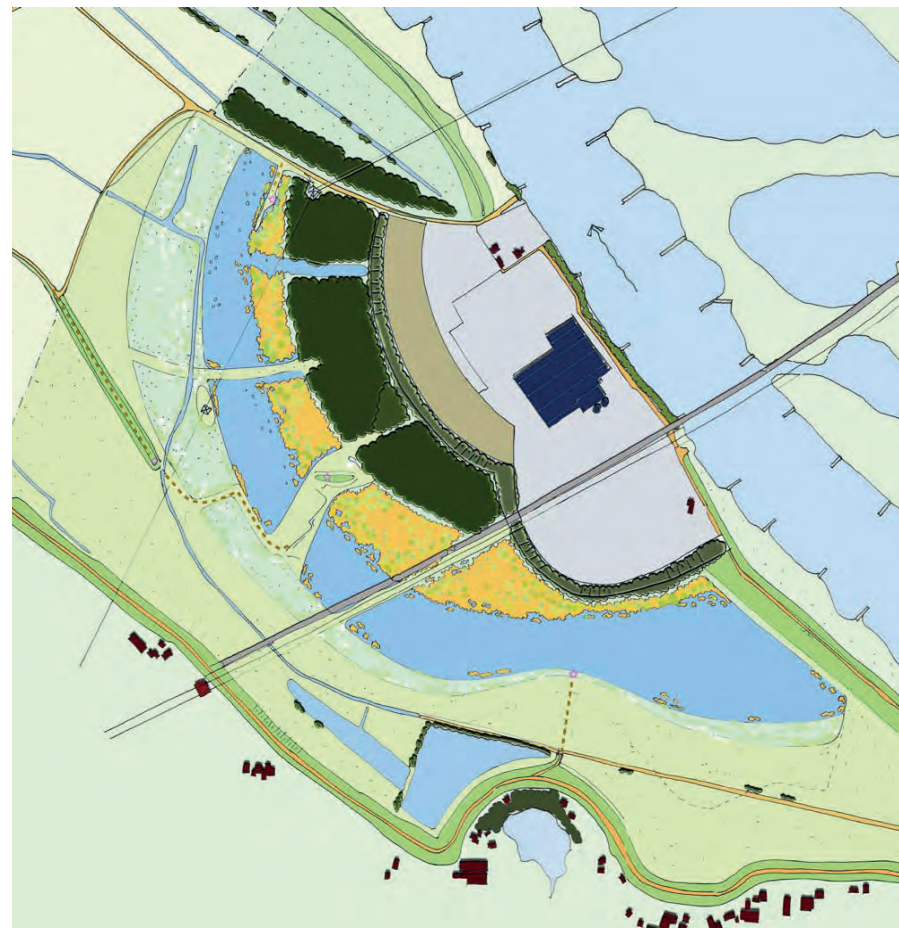
Figuur 24: Plankaart van het inrichtingsplan Angerensche en Doornenburgsche Buitenpolder. (Bron: Milieueffectrapport Angerensche en Doornenburgsche Buitenpolder, Lieveense, 7 maart 2017)
